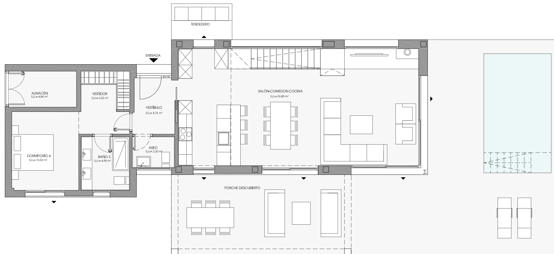
PLANTA BAJA
